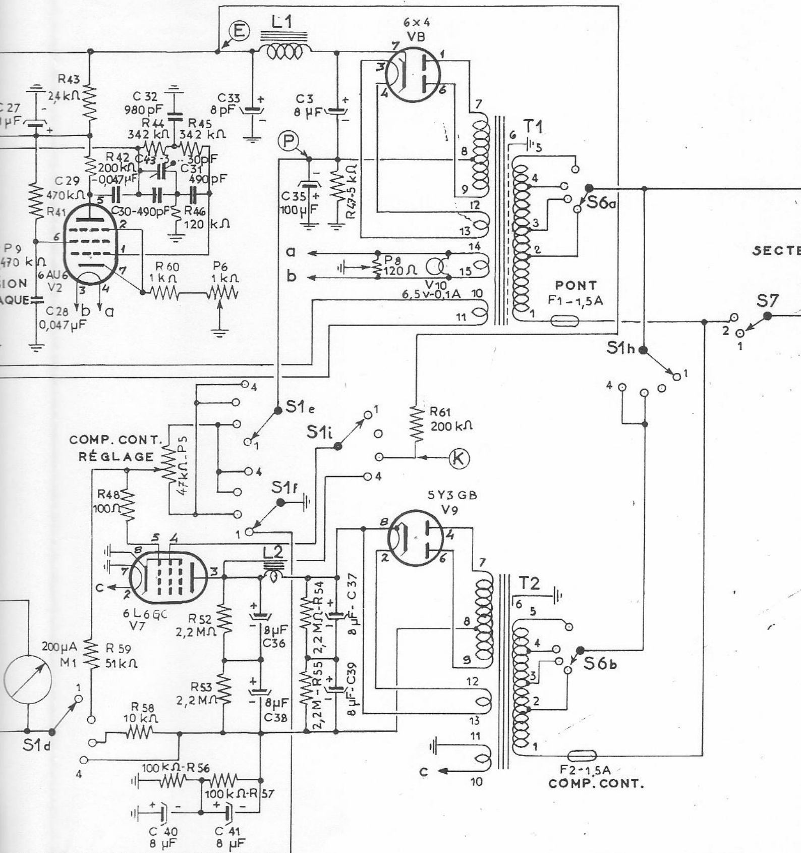
PONT D'IMPÉDANCES 626 B MÉTRIX. SCHÉMA DE PRINCIPE
